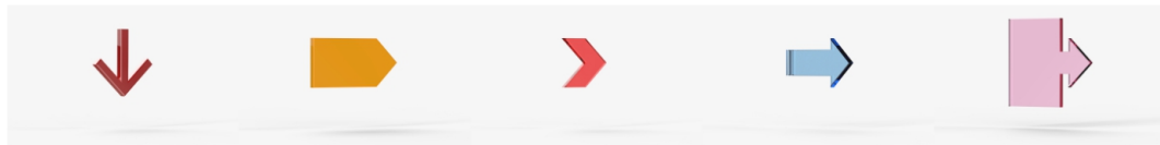
Arrow_Back_C
