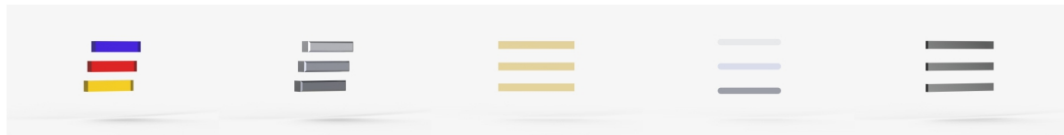
List_Group_B
