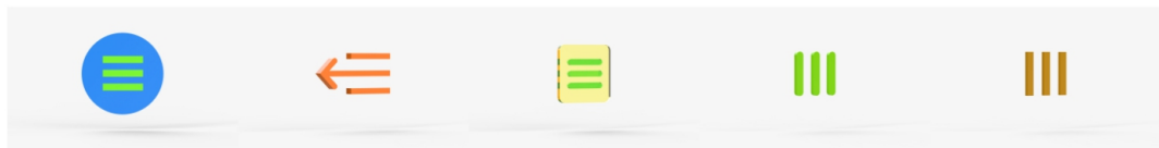
Icon_B_2
