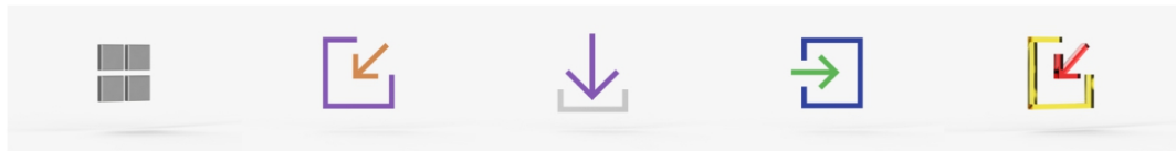
Icons_View_C
