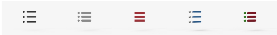
List_A
