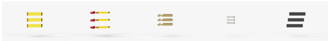
List_B_2
