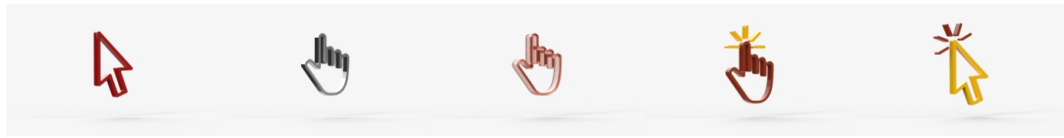
Icon_Cursor_B_1_01
