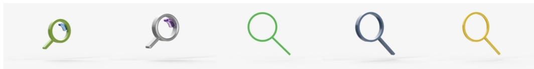
Search_2_B
