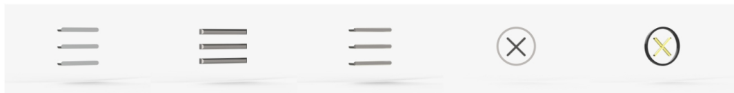
Menu_B_2
